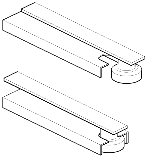
Sicherheitsbeschlag mit Pilzzapfen
