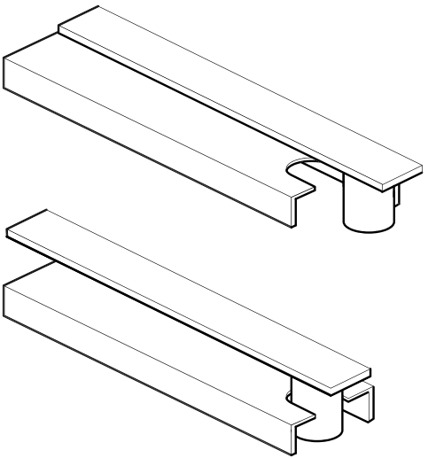
Standardbeschlag mit Rollzapfen
